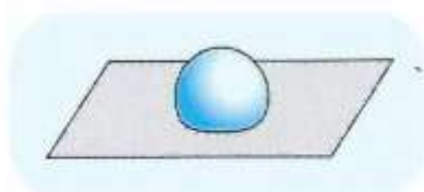
Etalement d'une goutte d'eau
